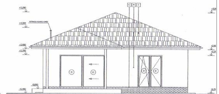
POHĽAD JUHOZÁPADNÝ
